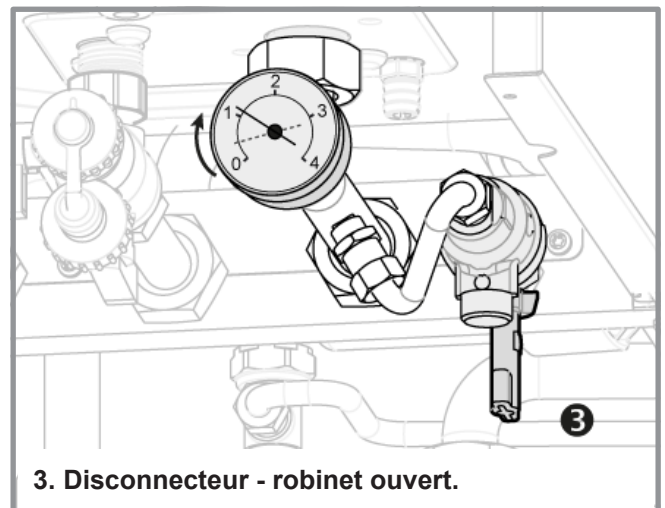
figure 5 - Remise en pression du circuit chauffage
